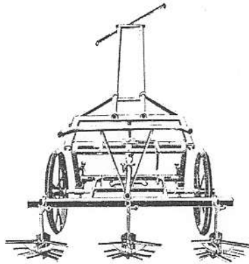
Umstellung der Deichsel für zweispänniges Arbeiten
