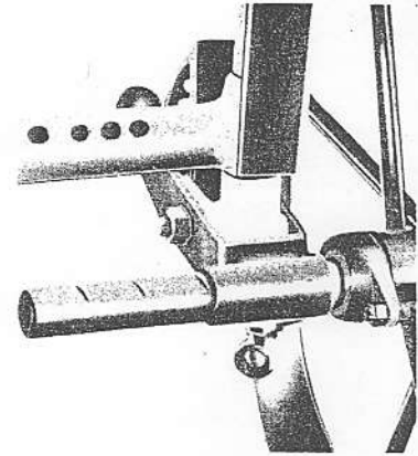
Bei Einstellen auf enge Spur keine vorstehende Achsstummel. Achsschenkel sind den Reihenweiten entsprechend markiert.
