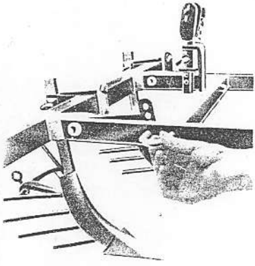
Flaches Zudecken und Hochhäufeln durch Schnittwinkelverstellung und Zinkenverstellung an den Häufelkörpern
