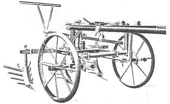
Ausrüstung B – Zudeck- und Häufelgerät Reihenweiten: wie beim Pflanzlochen
