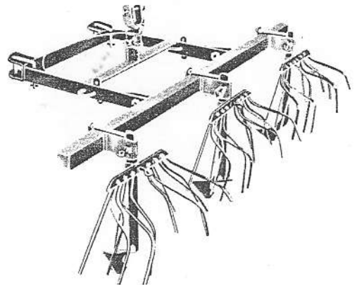
Ausrüstung C – Kartoffelhackeinrichtung mit Unkrauttriegeln
