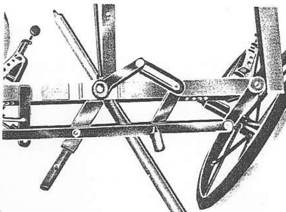
Umstellung von der Autosteuerung zur kombinierten Auto- und Rahmensteuerung durch einfaches Umstecken eines Bolzen
