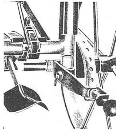
Tiefgangregulierung durch Einzelhöhenverstellung der Laufräder
